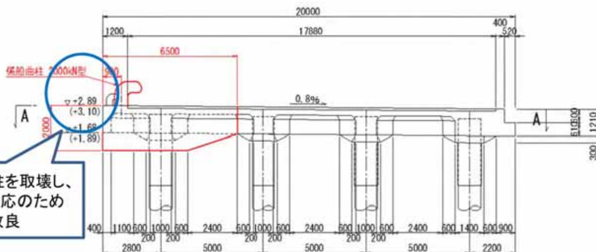
-断面図-
