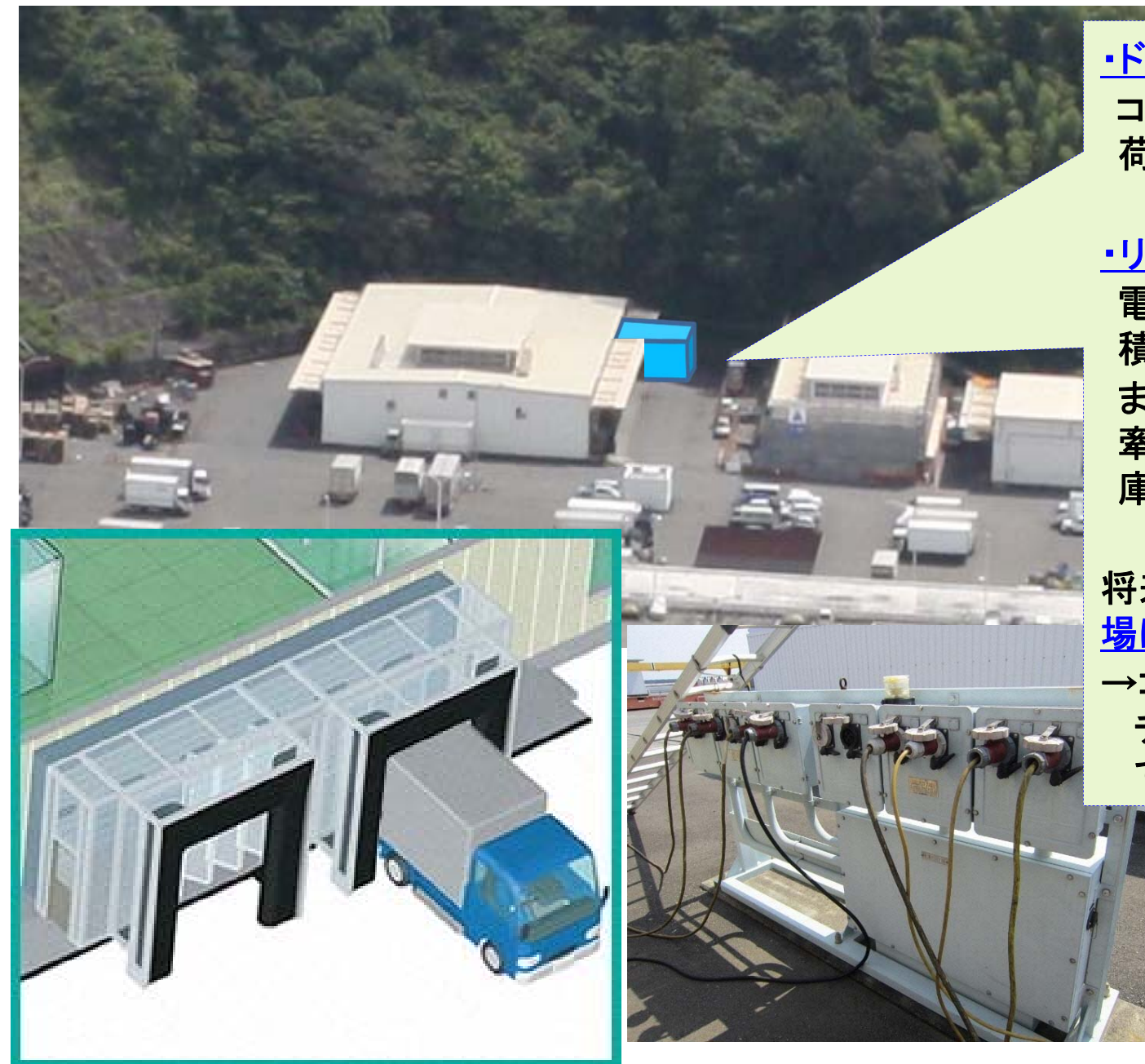
リーファーコンテナプラグ(イメージ)
