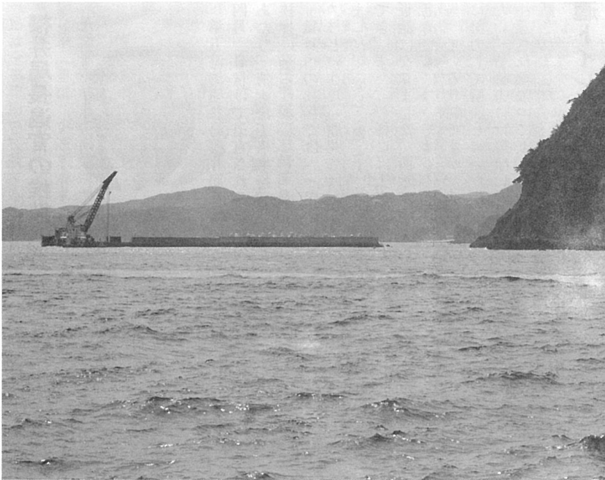
下田港：建設中の沖防波堤
