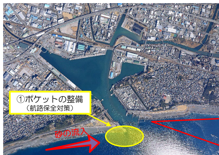
<田子の浦港の事業箇所>
