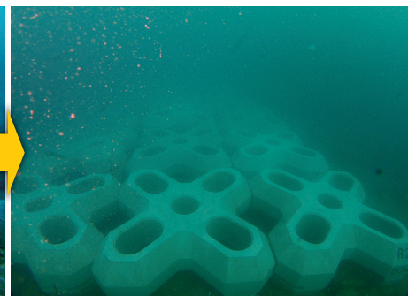
被覆ブロックの据付後 (2021年3月)
